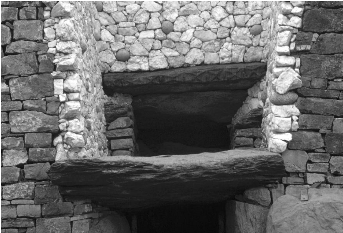
Passage Tomb , den långa gången in till kammaren har för det yttre partiet en parallell gång som löper ovanför den ordinarie gången, vilken släpper in solljus ända in till kammaren vid vintersolståndet. "Newgrange", Meath, Irland.
